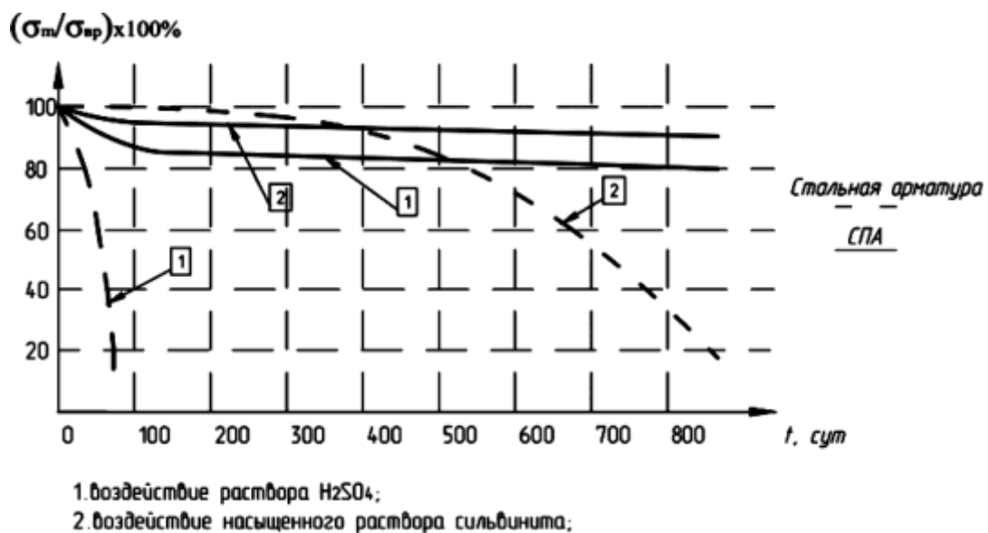
Рис. 3. Сравнительный анализ стойкости высокопрочной стальной и стеклопластиковой арматуры в агрессивных средах.
